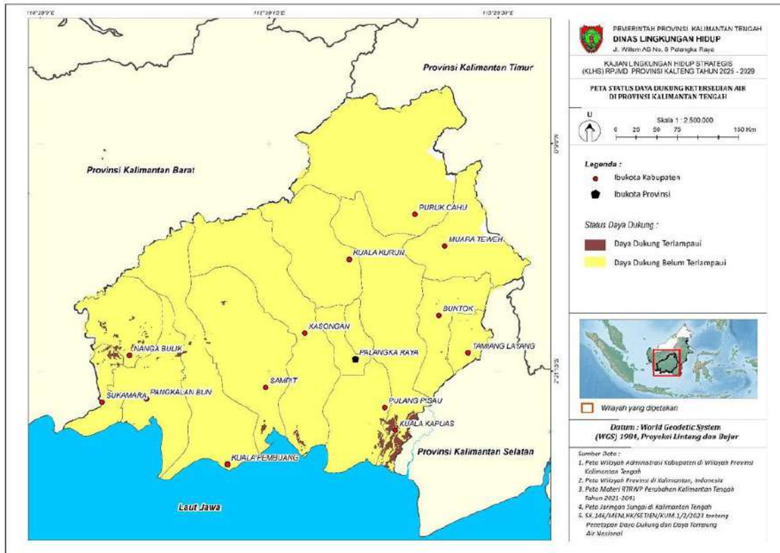
Gambar 2.1.11 Peta Status Daya Dukung Penyediaan Air Kalimantan Tengah
