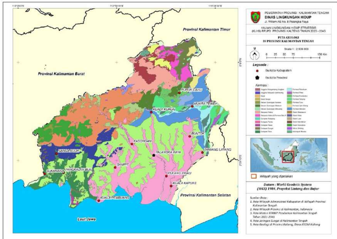
Gambar 2.1.3 Peta Persebaran Formasi Geologi di Kalimantan Tengah
