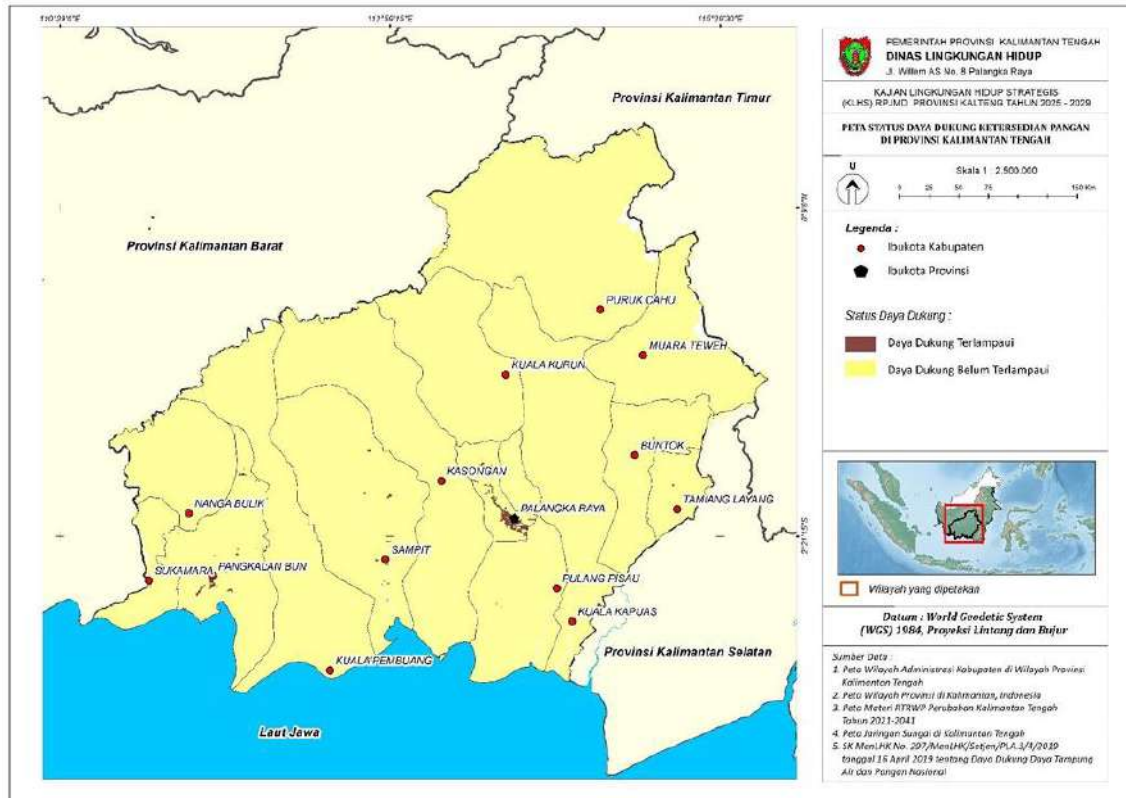
Gambar 2.1.12 Peta Status Daya Dukung Penyediaan Pangan Kalimantan Tengah
